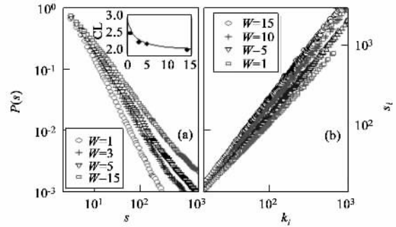
图 1 (a)网络结点强度的概率分布 P(s) , 模拟结果遵从幂函数律行为 s^{-\alpha} . 在右上角的嵌入小图中, 实心圆显示数据拟合所得到的 \alpha 值, 曲线显示解析表达式 \alpha = 2 + m/(m + 2W) . 这里的模拟数据是对于大小为 N = 5000 的 20 个网络的平均结果; (b) 在不同参数 W 下, 结点强度 s_i 作为结点连接度 k_i 的函数(纵横坐标双对数标度). 数据的线性拟合对于 W = 1, 5, 10, 15 , 得到的斜率分别为 1.04, 1.17, 1.25, 1.30, 从而证实强度与连接度之间的幂函数律关联 s \sim k^\beta
