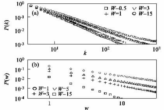
图 2 (a)网络结点连接度的概率分布 P(k) \sim k^{-\gamma} (b) 网络连边权重的概率分布 P(w) \sim w^{-\eta} . 模拟数据是对于大小为 N = 5000 的 20 个网络的平均结果
